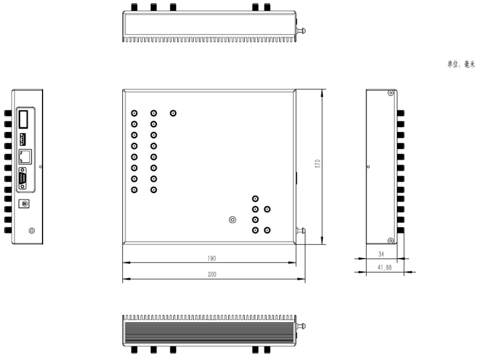
图 2 Venus Lite 系列产品外观和结构尺寸图
