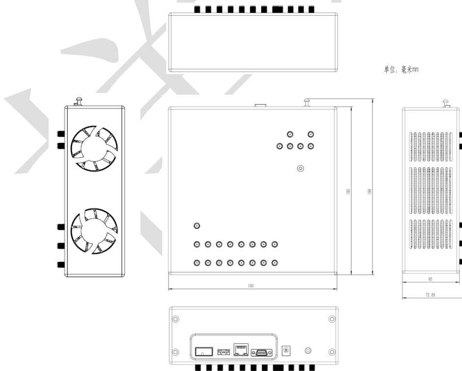
图 3 Venus Lite-T 系列产品外观和结构尺寸图
